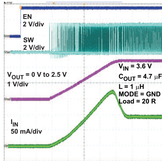
t - Time - 20 µs/div
