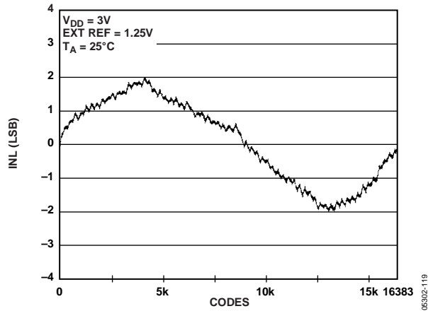
Figure 20. INL AD5648-1
